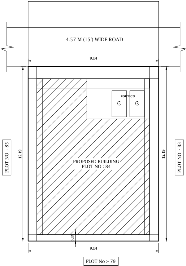
SITE PLAN 1:100
