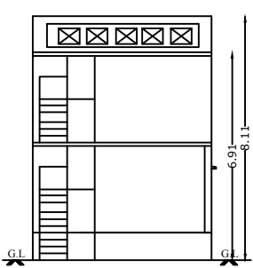
ELEVATION
