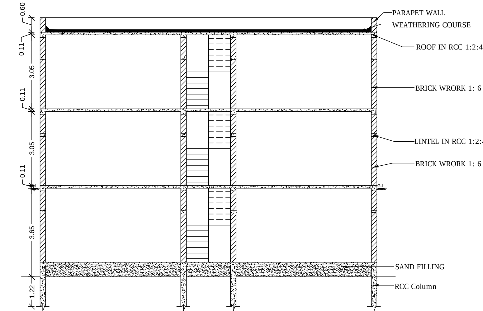
SECTION A-B
