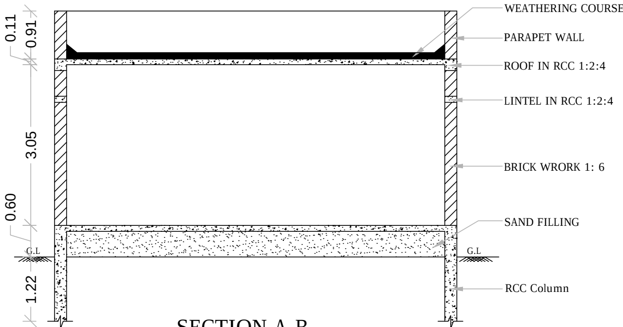
SECTION A-B
