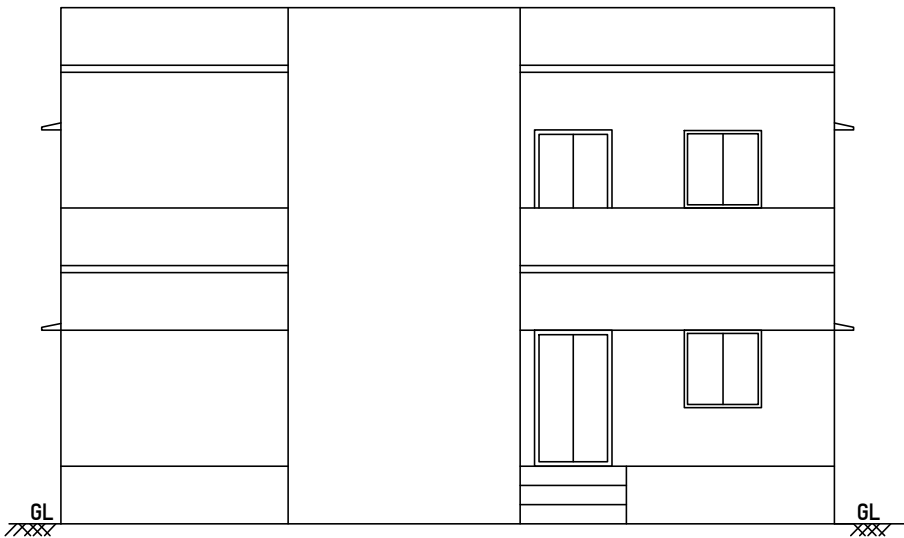
ELEVATION
