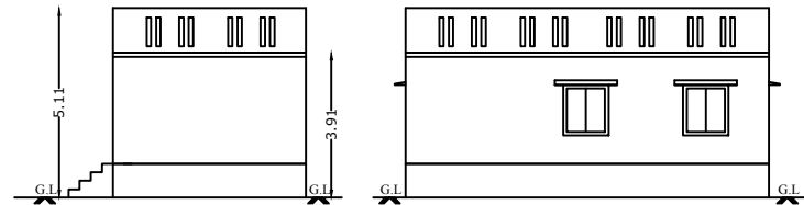
ELEVATION
