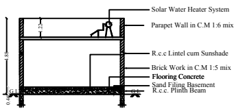
SECTION A-B
