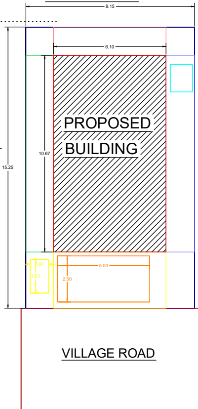
SITE PLAN 1:100
