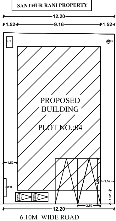
SITE PLAN ( SCALE: 1:100)
