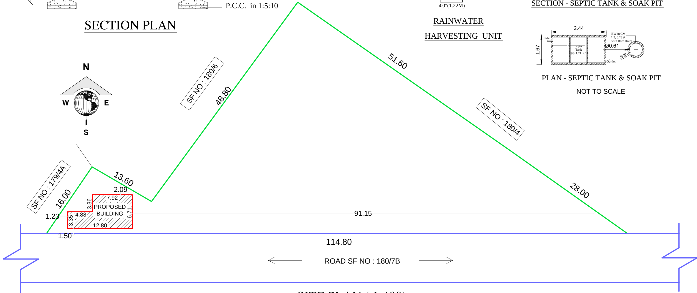
SITE PLAN ( 1:400)
