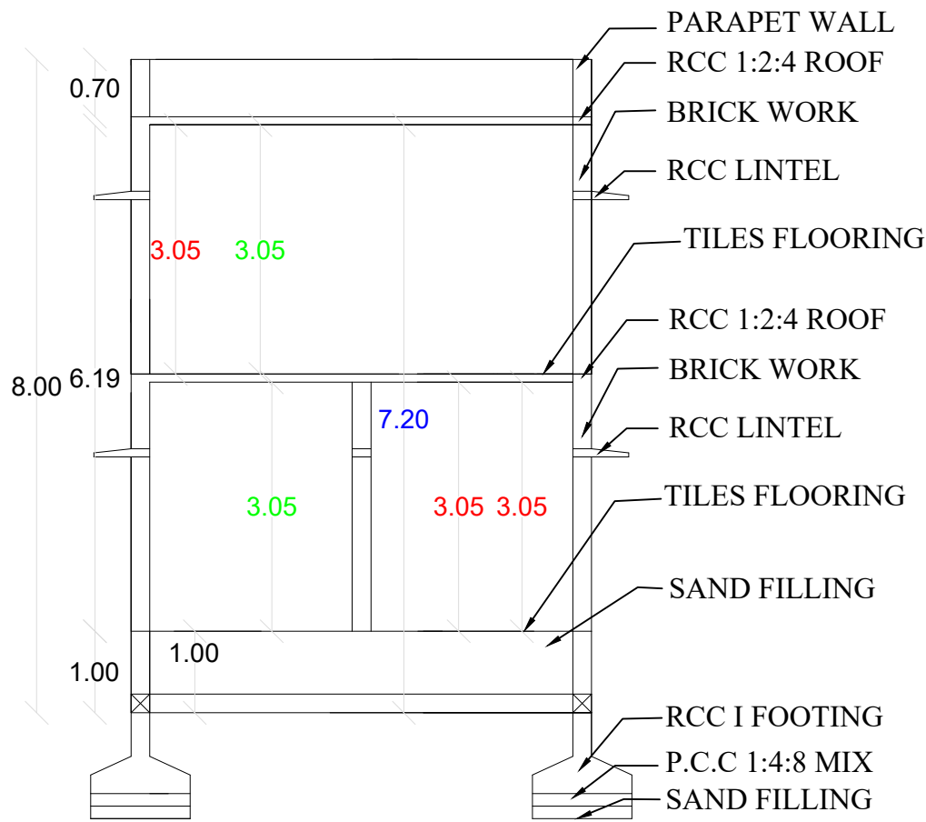
SECTION A-B
