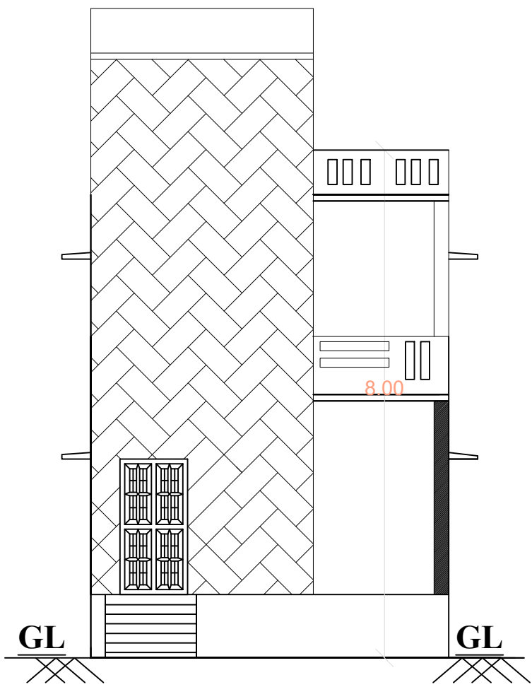
ELEVATION
