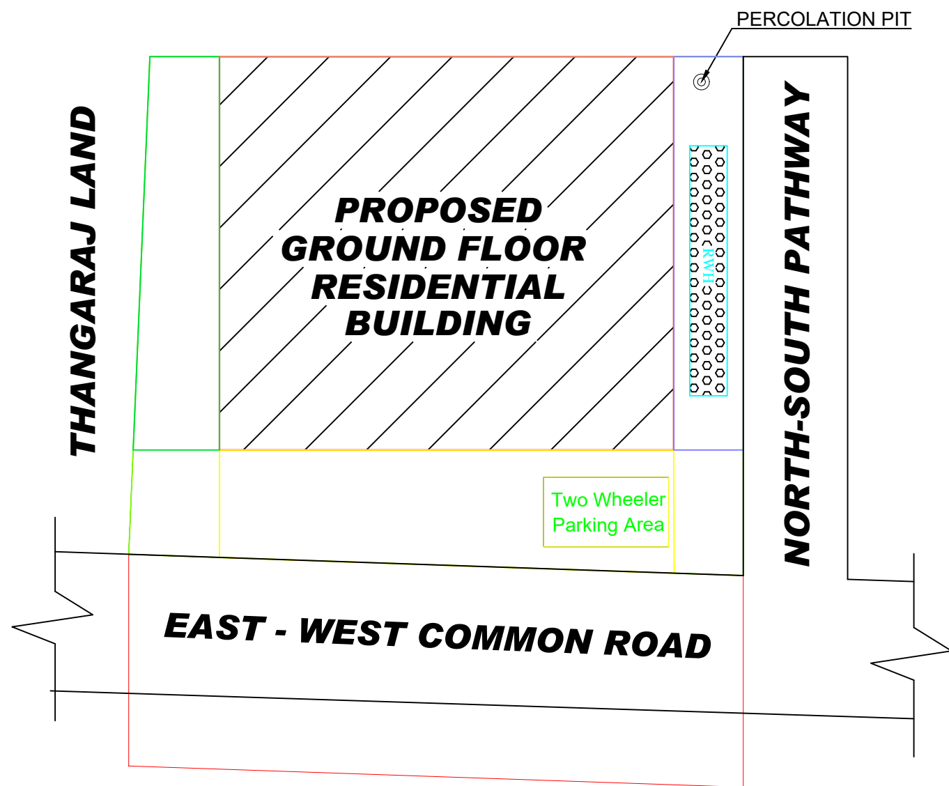
SITE PLAN (SCALE: 1:1)
