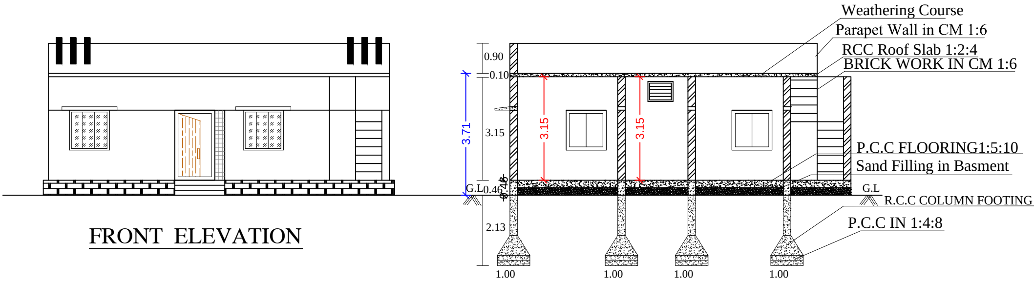
SECTION - A-B
