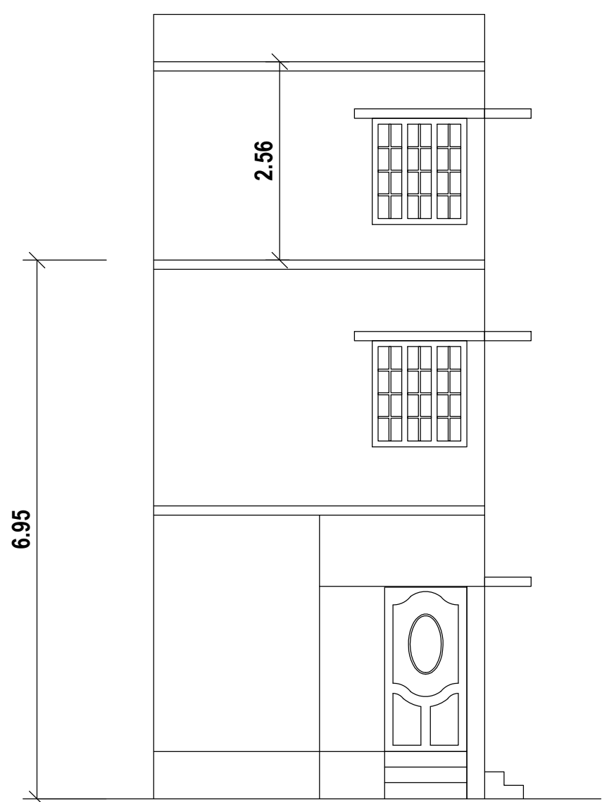
ELEVATION
