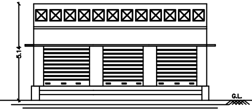
ELEVATION
