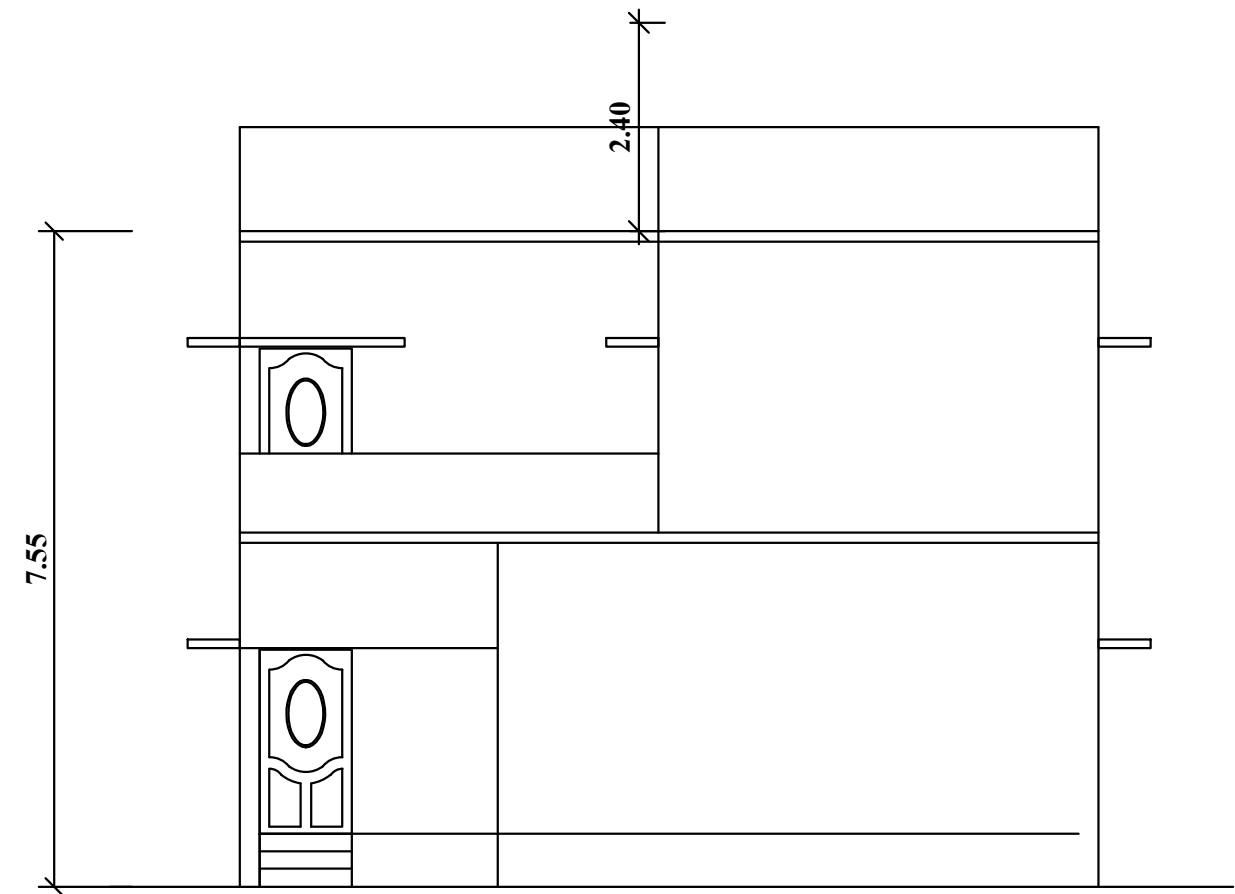
ELEVATION
