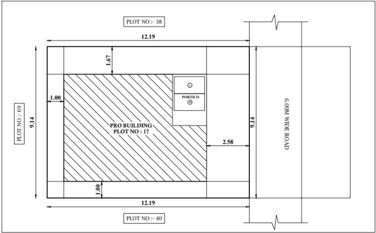
SITE PLAN 1:100
