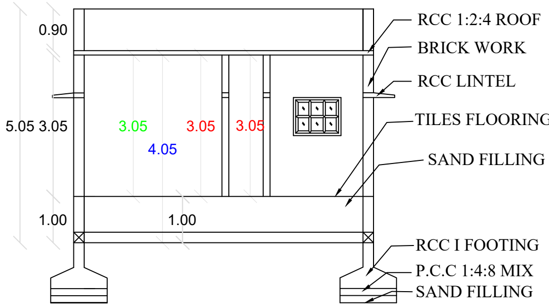
SECTION A-B
