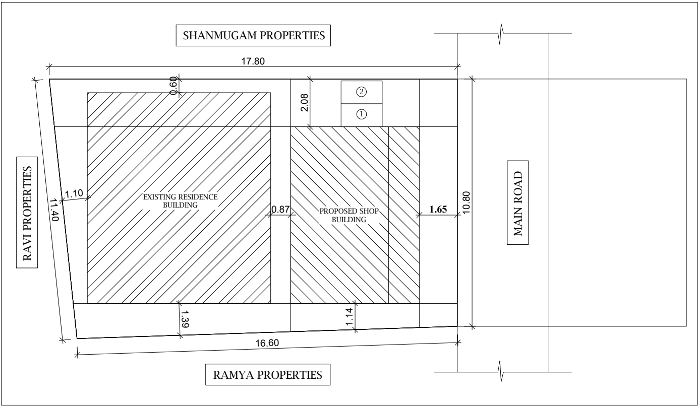
SITE PLAN 1:100
