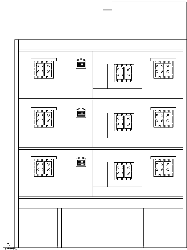
ELEVATION
