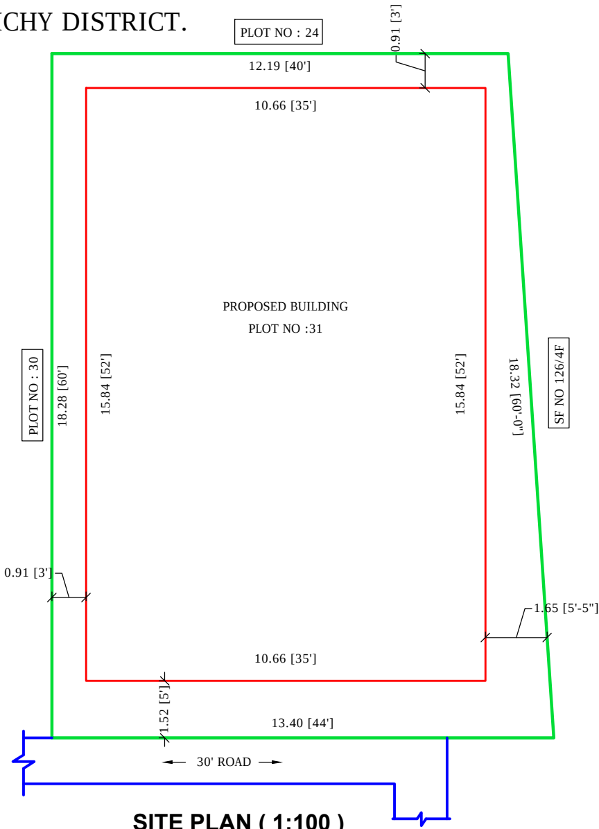
SITE PLAN ( 1:100 )
