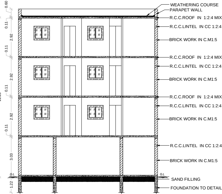
SECTION A-B
