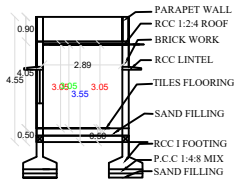
SECTION A-B
