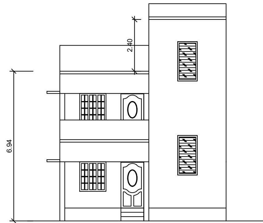
ELEVATION
