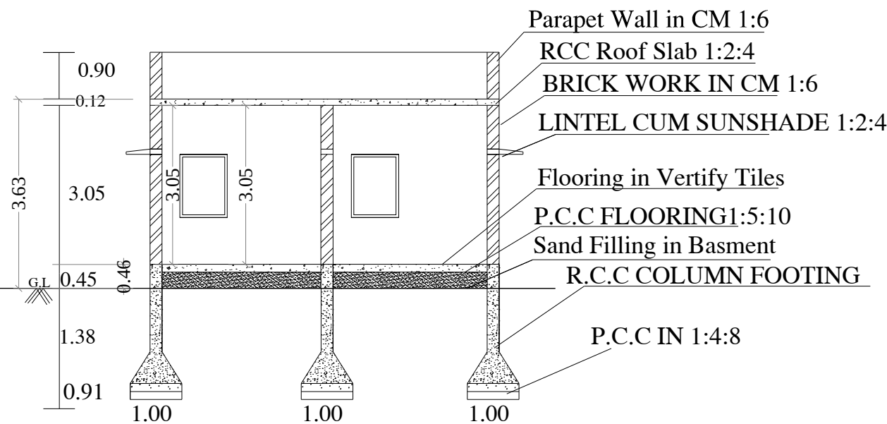
SECTION - AB
