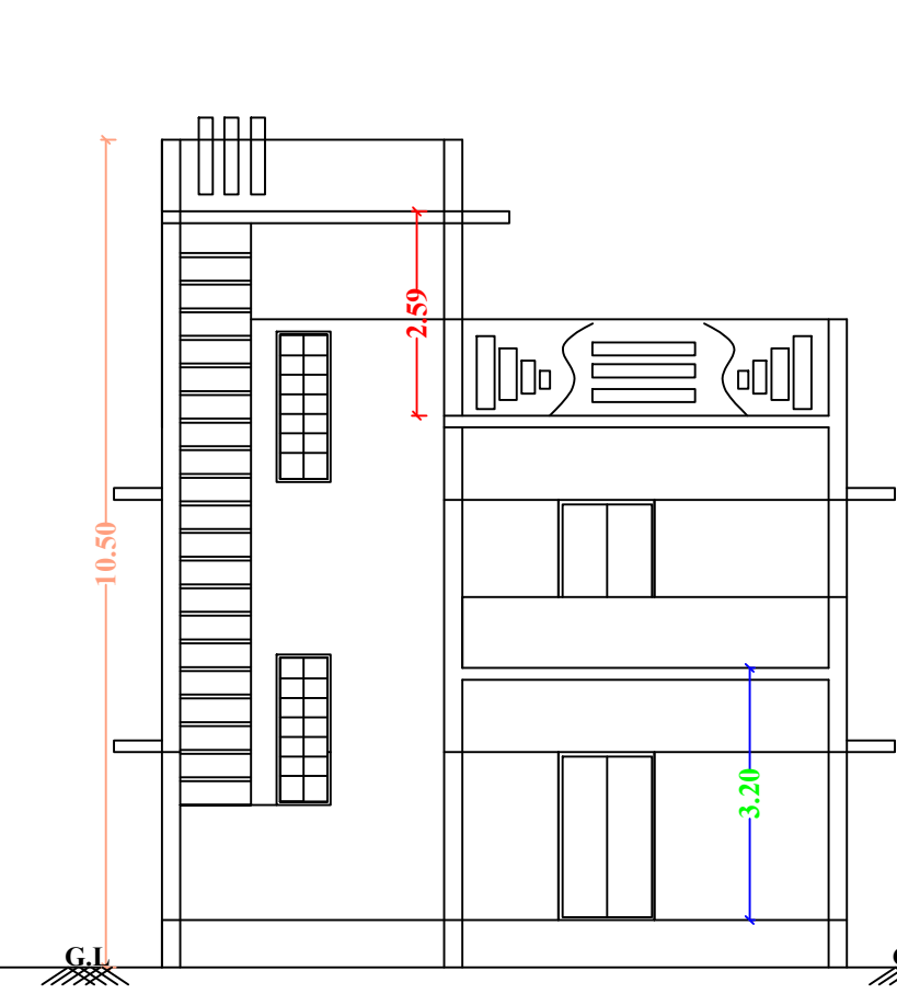
ELEVATION
