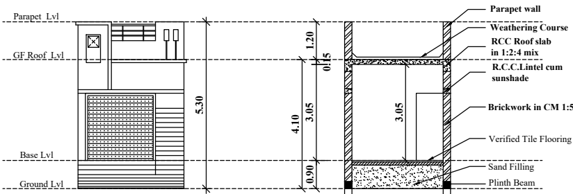
ELEVATION
