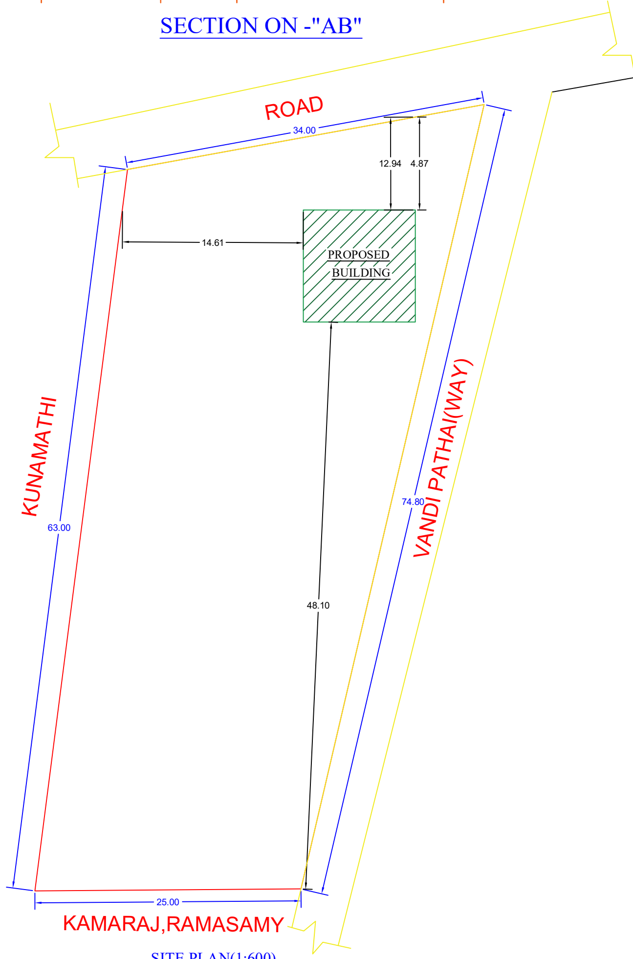
SITE PLAN(1:600)
