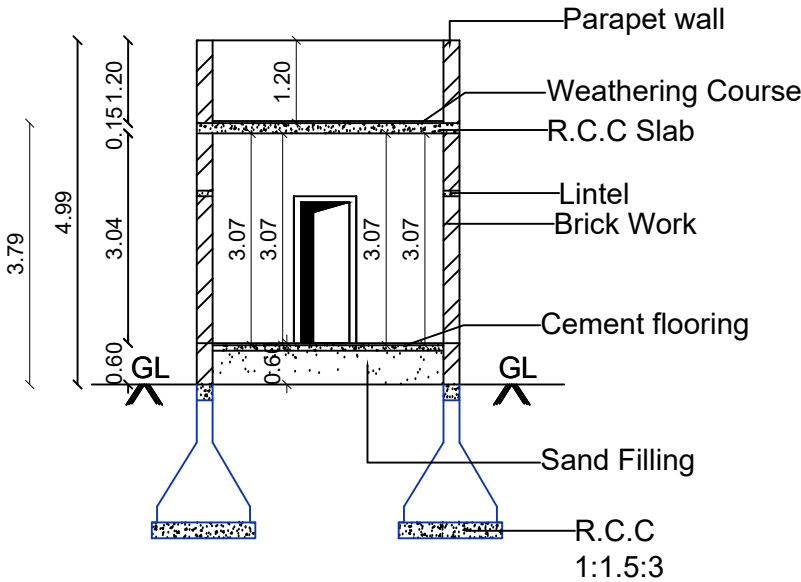
SECTION ON'AB'
