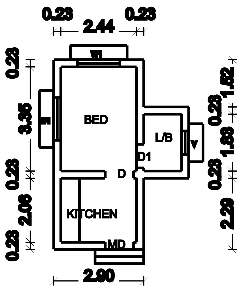
G.F PLAN
