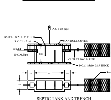
SECTION - AB
