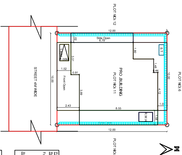
SITE PLAN (SCLAE - 1:100)
