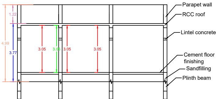
SECTION - AB
