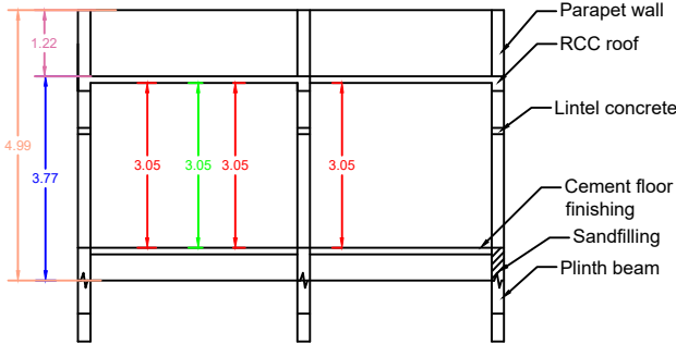
SECTION - AB
