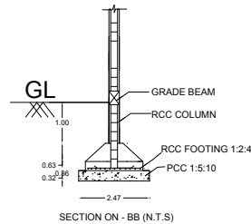
SECTION ON - BB (N.T.S)
