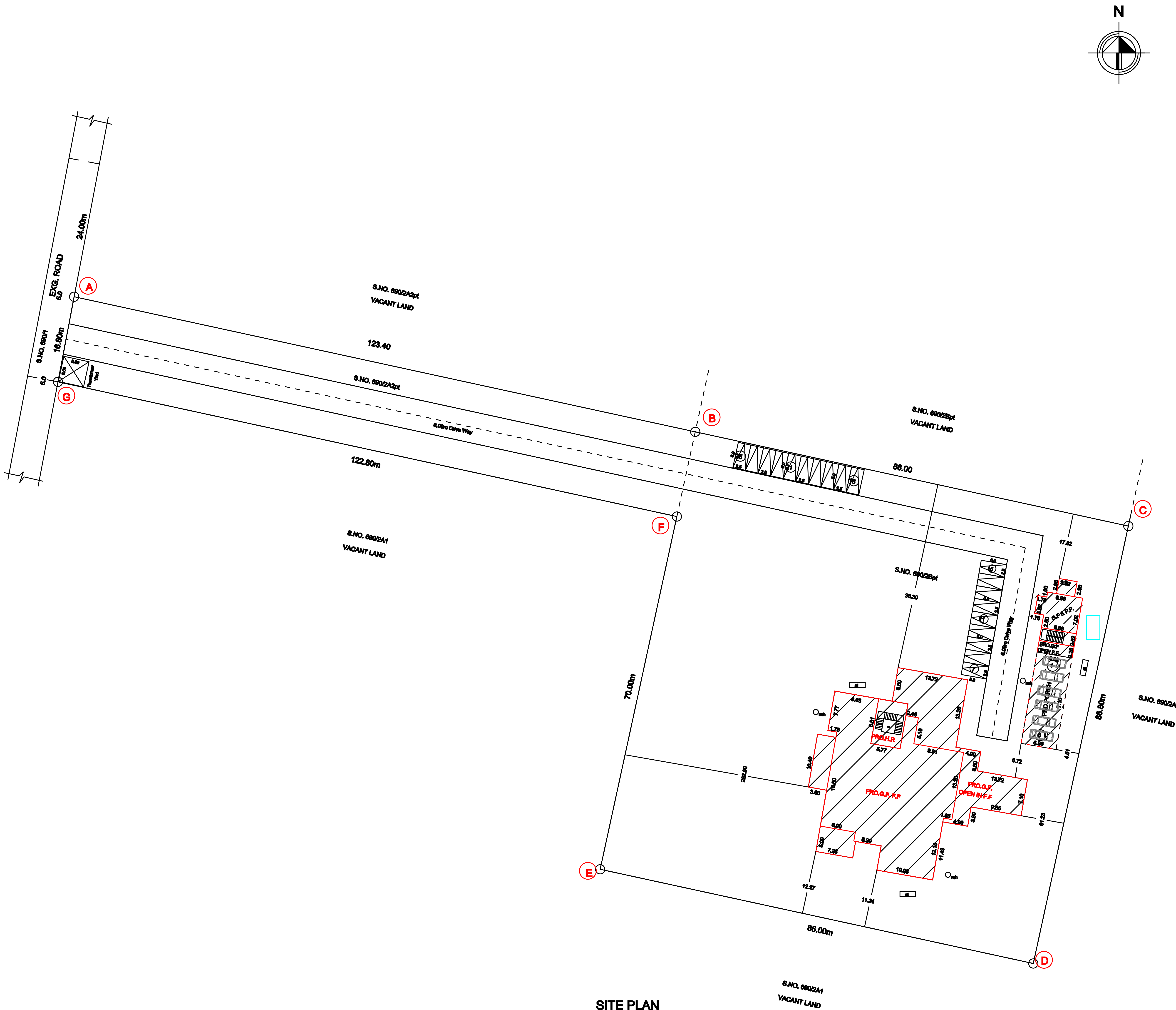
SITE PLAN SCALE 1:400
