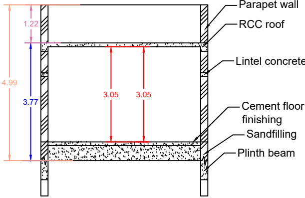
SECTION - AB
