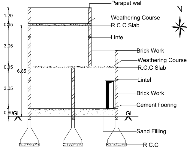
SECTION ON'AB'
