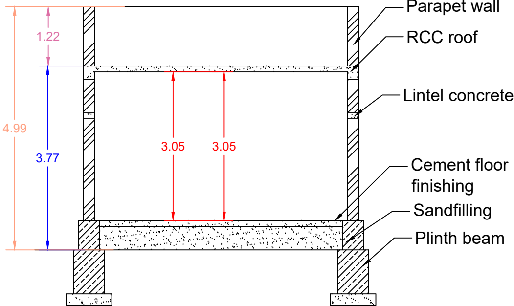
SECTION - AB
