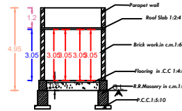
SECTION A-B
