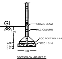
SECTION ON - BB (N.T.S)
