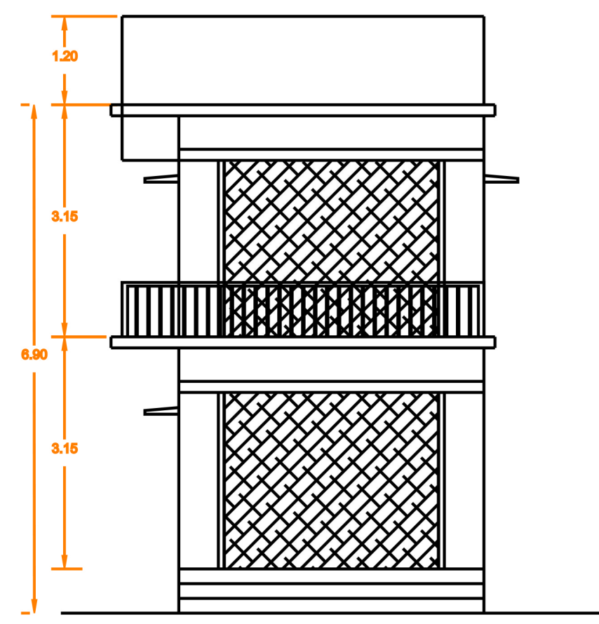
ELEVATION - A
