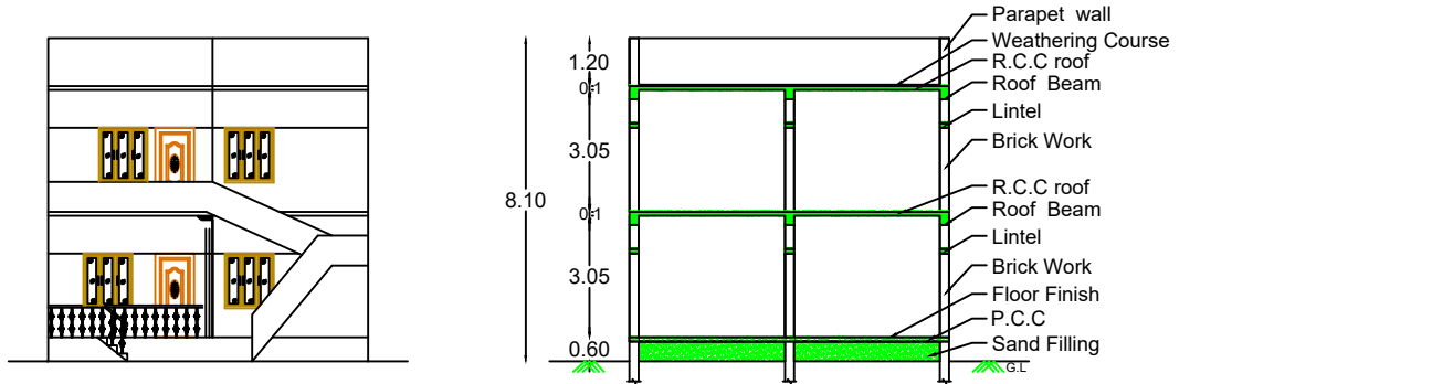
ELEVATION
