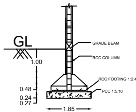
SECTION ON - BB (N.T.S.)
