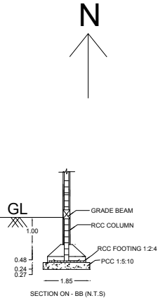
SECTION ON - BB (N.T.S)
