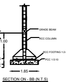
SECTION ON - BB (N.T.S.)
