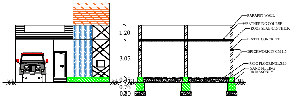
ELEVATION
