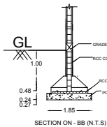
SECTION ON - BB (N.T.S.)
