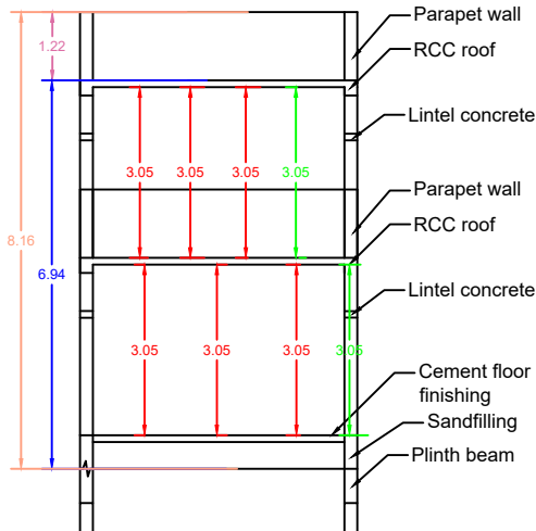
SECTION - AB
