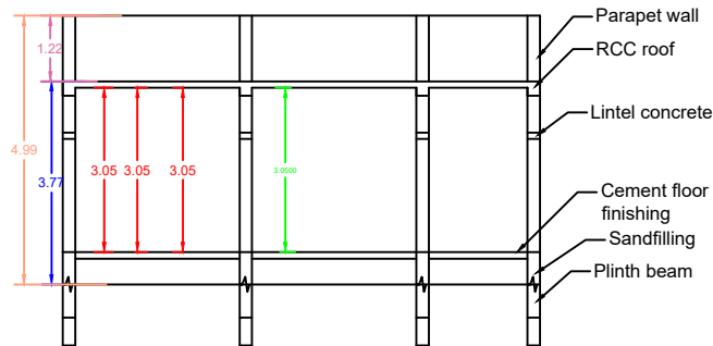
SECTION - AB
