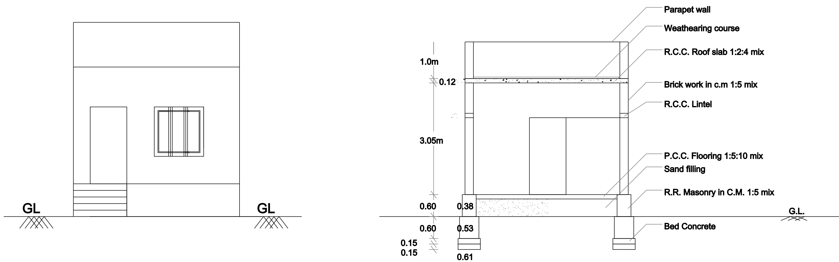
ELEVATION
