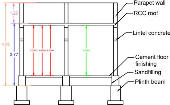
SECTION - AB
